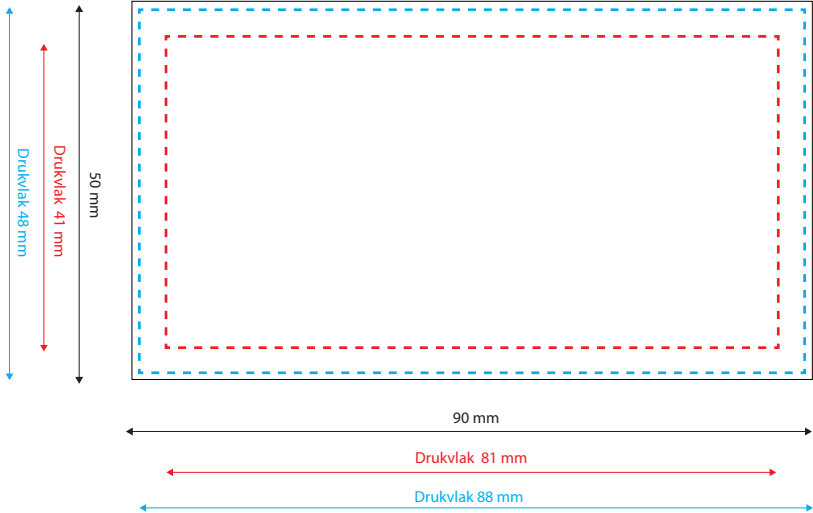
Zijde 2
